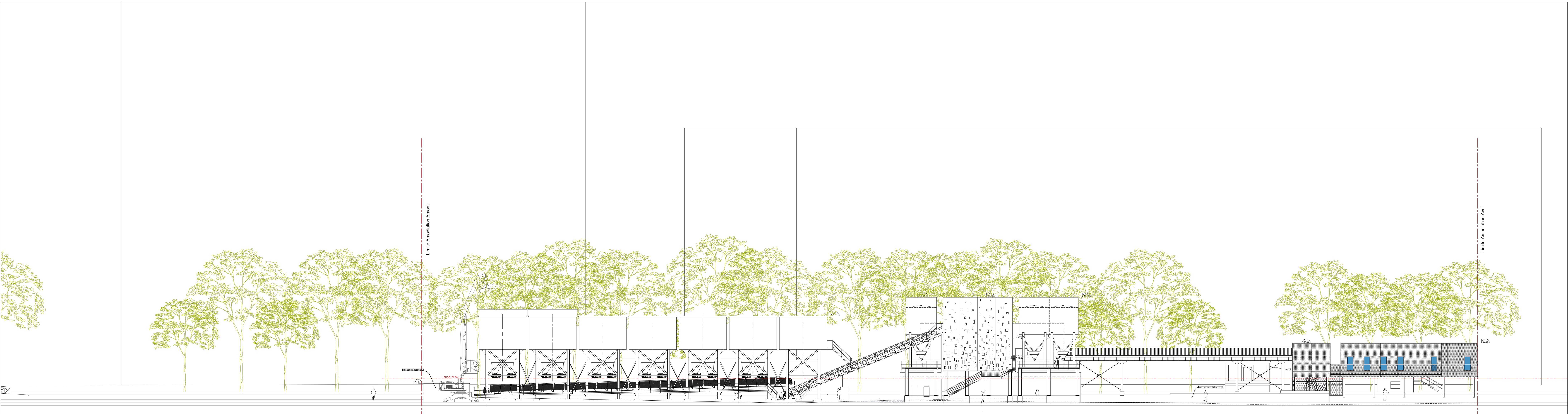
Façade 1.1 depuis la Seine sans clôture
